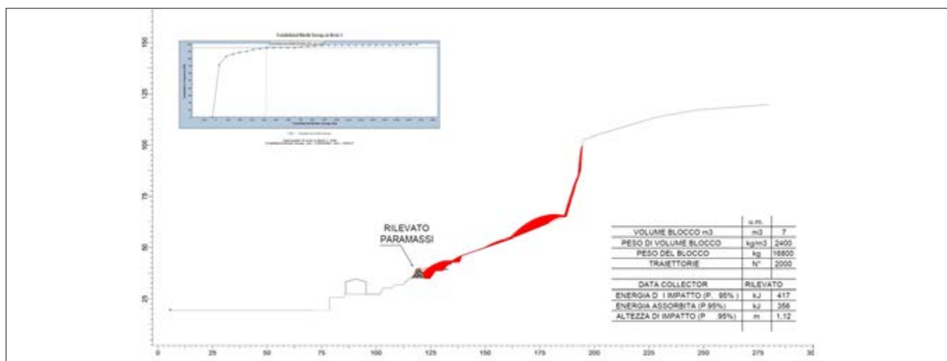
Figura 10. Simulazione caduta massi (Software RocFall) - Mappa Fs locale Versante-Barriera (Software SSAP-2018)
