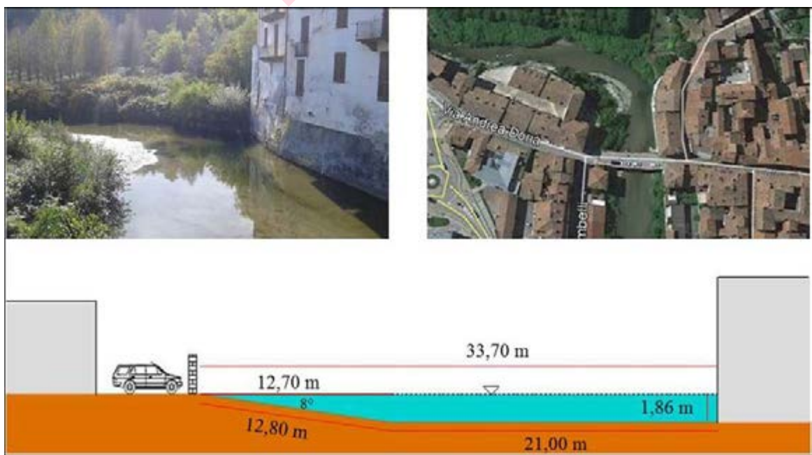
Figura 11. Ubicazione e schema semplificato della sezione C2, in corrispondenza dell'ansa fluviale del T. Cevetta, a circa 30 m dal ponte che collega via Doria con via Marenco
