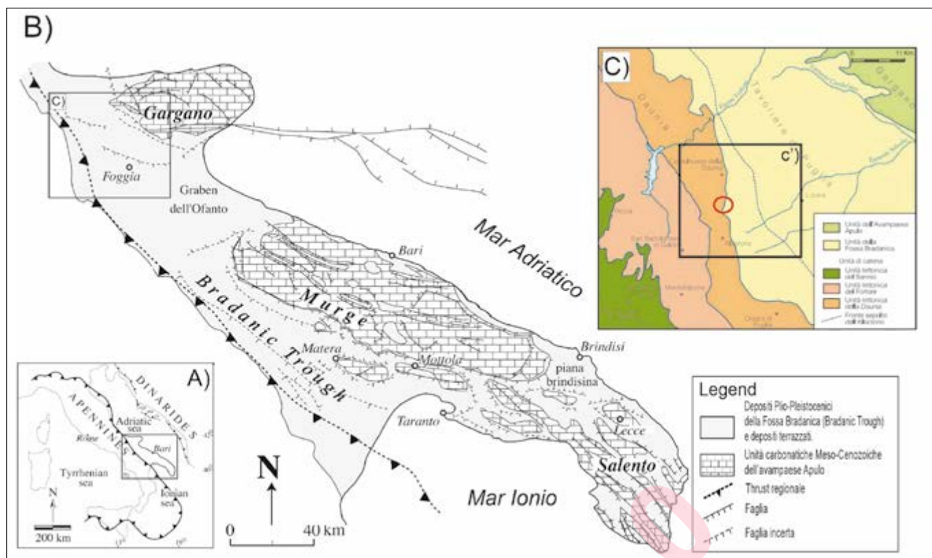
Figura 1. A) Inquadramento dell'area studio. B) Schema geologico strutturale della Regione Puglia, modificato da Pieri et al. , 1997. C) Schema geologico strutturale dell'Apennino Dauno, con il cerchio in rosso è riportata l'ubicazione dell'area studio. (c') Estensione del Foglio 407 del Progetto CARG alla scala 1: 50.000
